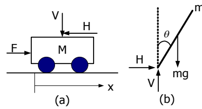
圖 9. 車與倒單擺示意圖
