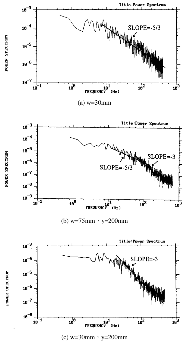
圖 7. 二維網格紊流之速度微擾分析。U=1.2m/s, d=1.0mm
