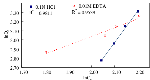
圖 8. 土壤中鋅之 Freundlich 模式
