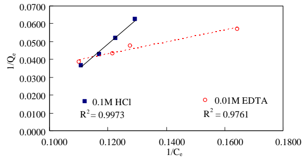
圖 7. 土壤中鋅之 Langmuir 模式
