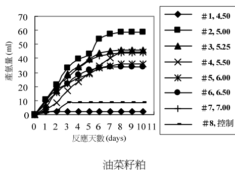
圖 1. 當油菜、油菜籽粕基質 COD 濃度為 20,000 mg/L 下，不同起始 pH 之累計產氫
