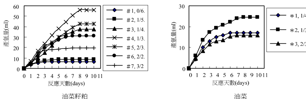
圖 6. 當油菜、油菜籽粕基質 COD 濃度為 20,000 mg/L，不同混合菌液/基質配比之累積產氫圖
