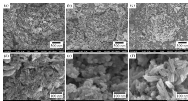
圖 3. 添加 (a, d) 葡萄皮、(b, e) 地瓜皮、(c, f) 柚子皮萃取物，合成奈米級氫氧基磷灰石，水熱處理溫度為 150 °C，水熱處理時間為 48 h，pH 值為 10 之 FE-SEM 照片 (倍率：×30000; ×200000)
