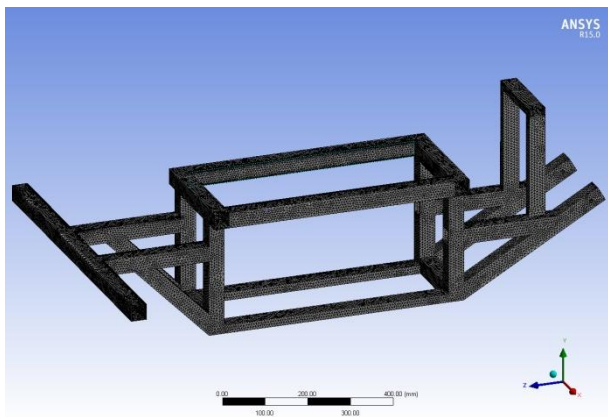
圖 6. 整體的車架網格顯示
