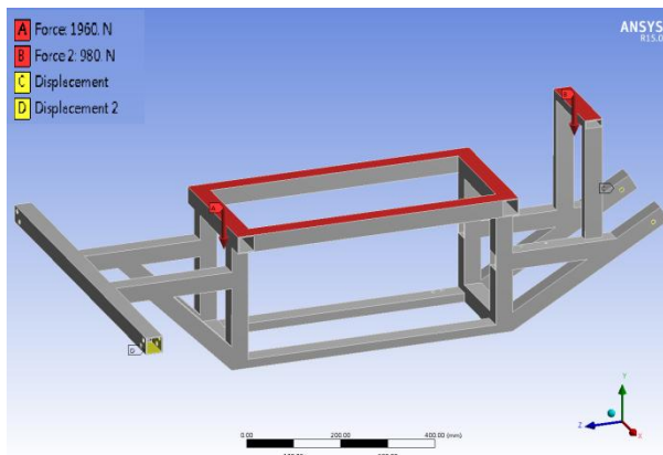
圖 7. 車架應力分析邊界條件
