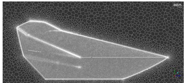
圖14. 中心截面的網格
