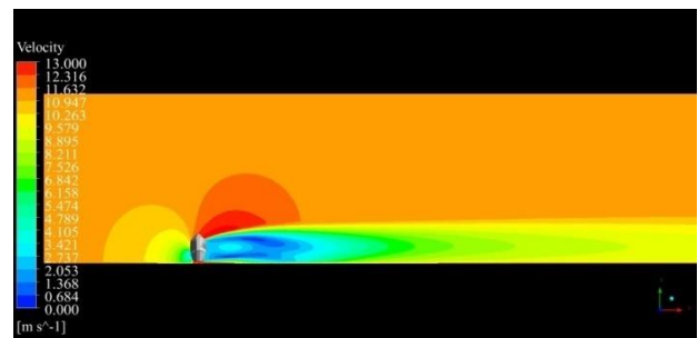
圖 18. 車長一半處的截面速度場
