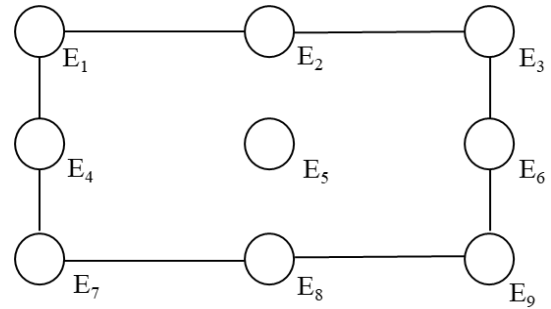
圖 10. 平均照度法 9 點量測法
