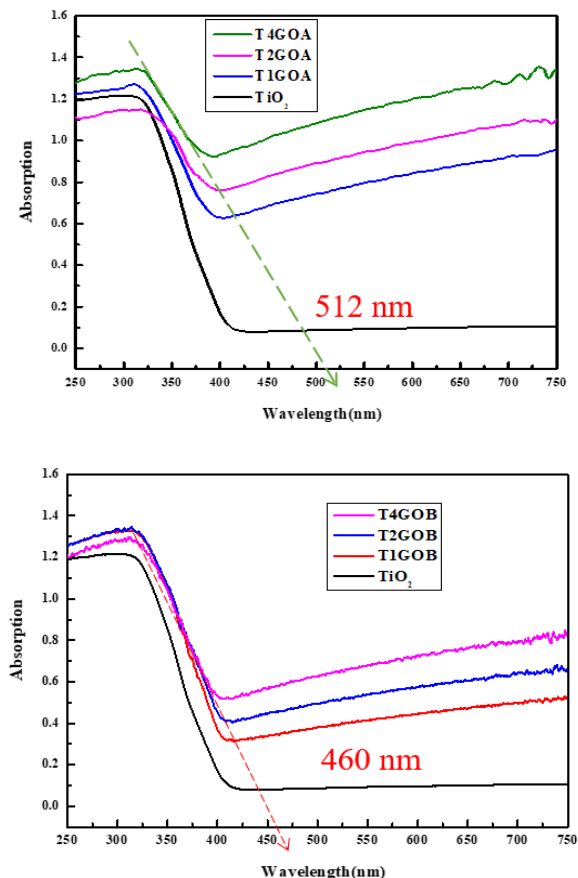
圖 8. 不同氧化石墨烯及比例改質 TiO 2 之 UV-Vis 圖譜
