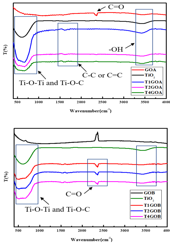
圖 7. 不同氧化石墨烯及比例改質 TiO 2 之 FTIR 圖譜
